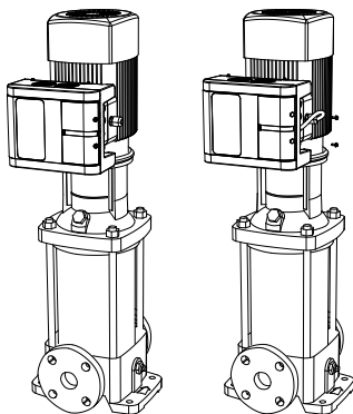
图 2-4-2 PDH30 安装操作
