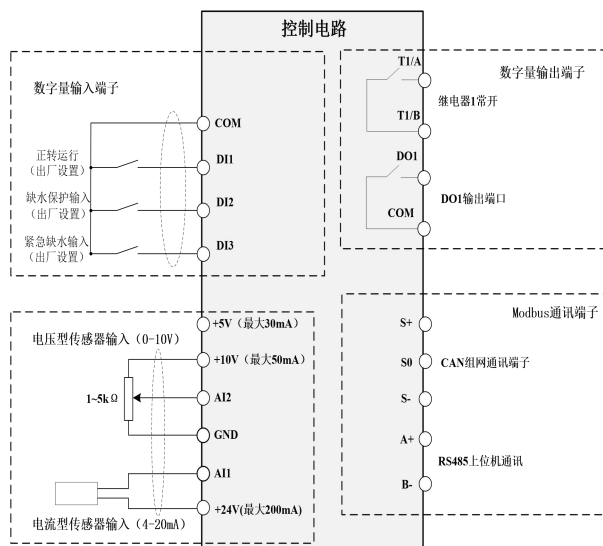
图 2-6-1 0.75kW-7.5kW 控制端子
