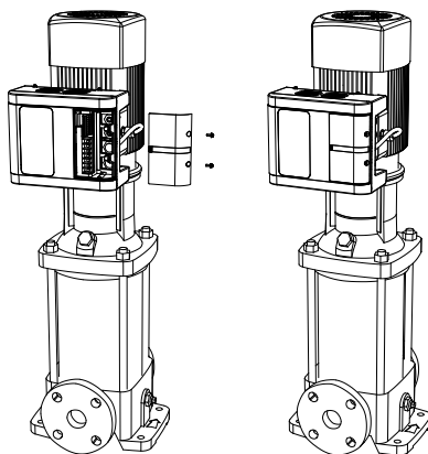
图 2-4-3 PDH30 安装操作
