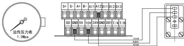
图 2-7-1 远程压力表接线图
