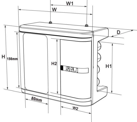
图 2-3-1 0.75kW-2.2kW 外形尺寸示意图
