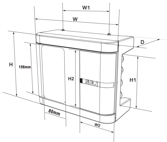
图 2-3-2 4kW-7.5kW 外形尺寸示意图
