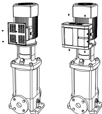
图 2-4-1 PDH30 安装操作
