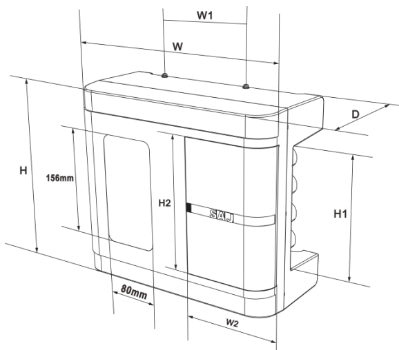
图 2-3-3 11kW-18.5kW 外形尺寸示意图
