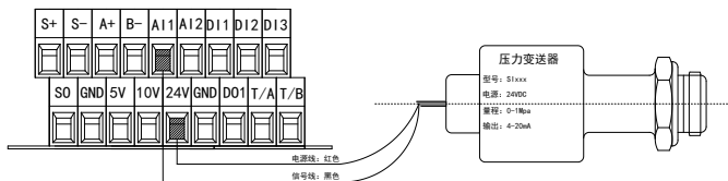
图 2-7-2 两线制压力变送器接线图
