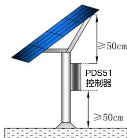
图 3-3-2 安装位置
