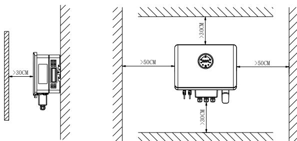
图 3-4-2 安装空间要求
