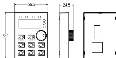
图 3-2-1 键盘尺寸图
