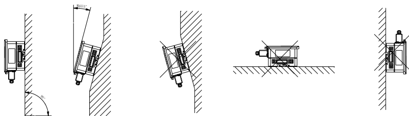
图 3-4-1 正确安装方向
