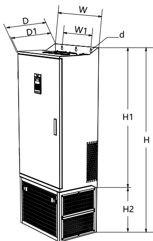
图 2-3-3 外形尺寸 3
