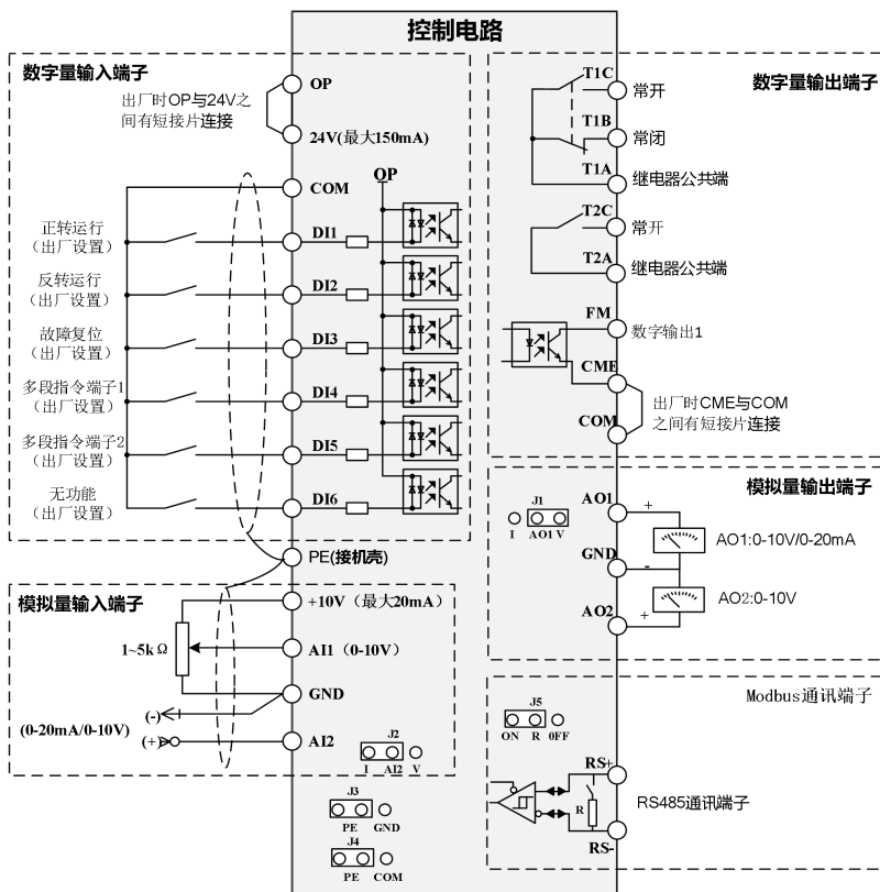
图 2-6-2 控制回路示意图 2
