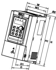
图 2-3-1 外形尺寸 1
