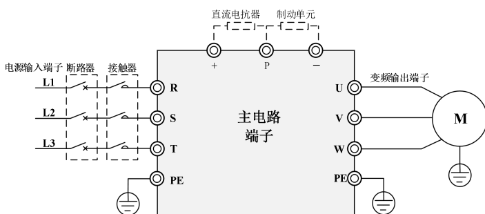
图 2-5-2 主电路端子示意图 2
