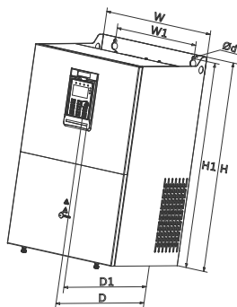
图 2-2-2 外形尺寸 2
