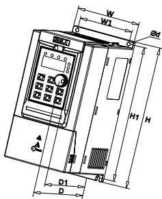
图 2-2-1 外形尺寸 1
